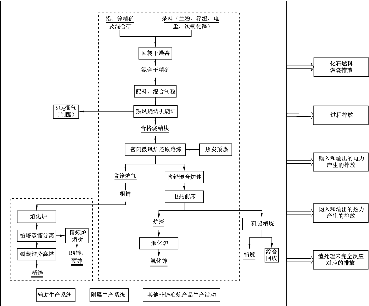
A.2 锌冶炼企业典型火法炼锌工艺温室气体排放核算边界示意图见图 A.2。
